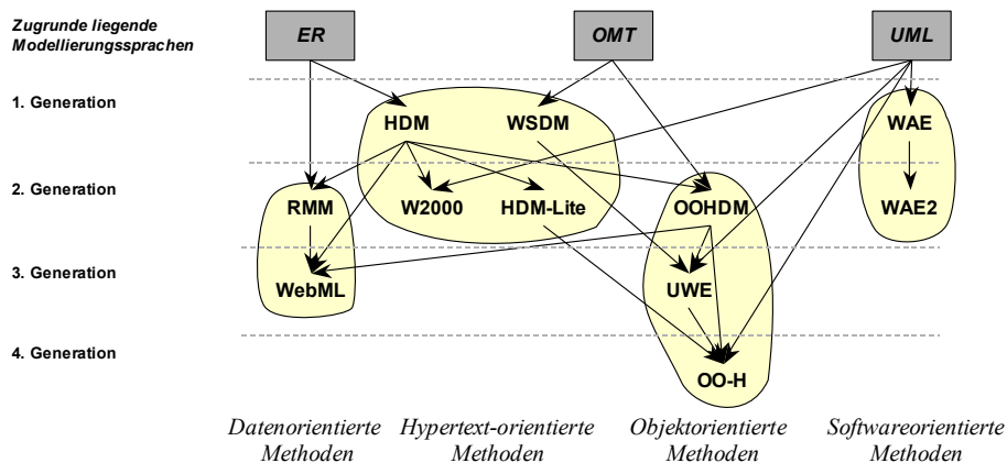
Abb. 3-13 Historische Entwicklung der Methoden zur Modellierung von Web-Anwendungen
