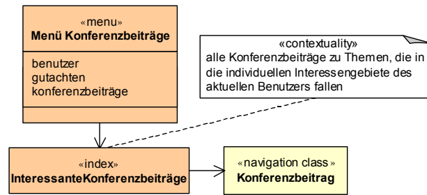
Abb. 3-11 Dynamische Adaptierung eines Index im Hypertext-Modell
