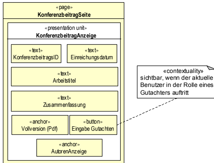
Abb. 3-12 Dynamische Adaptierung einer Seite im Präsentationsmodell
