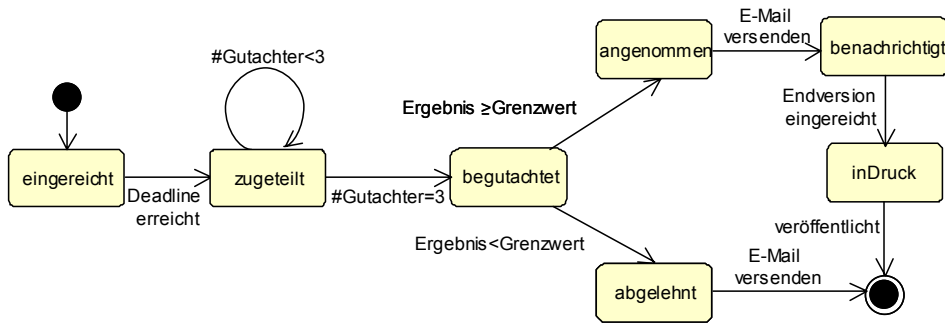
Abb. 3-6 Zustandsdiagramm für einen Konferenzbeitrag
