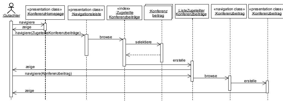
Abb. 3-10 Szenario aus dem Präsentationsmodell des Begutachtungssystems
